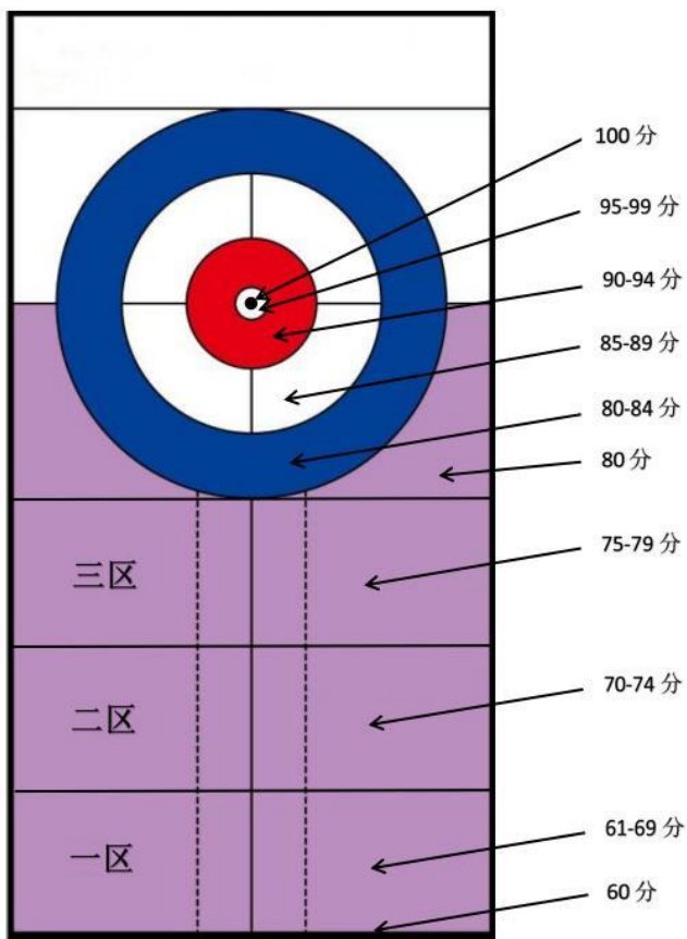
图 5-1 分值示意图
